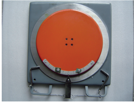
LASEROWY POMIAR ZBIEŻNOŚCI KÓŁ PRZEDNICH Z ZASTOSOWANIEM PRECYZYJNEJ OBROTNICZY (ZDĘCIE ŚRODKOWE) I UNIWERSALNEGO UCHWYTU GŁOWICY (Z PRAWY) UMOŻLIWIĄJĄCEGO KOMPENSOWANIE BICIA OBRĘCZY
