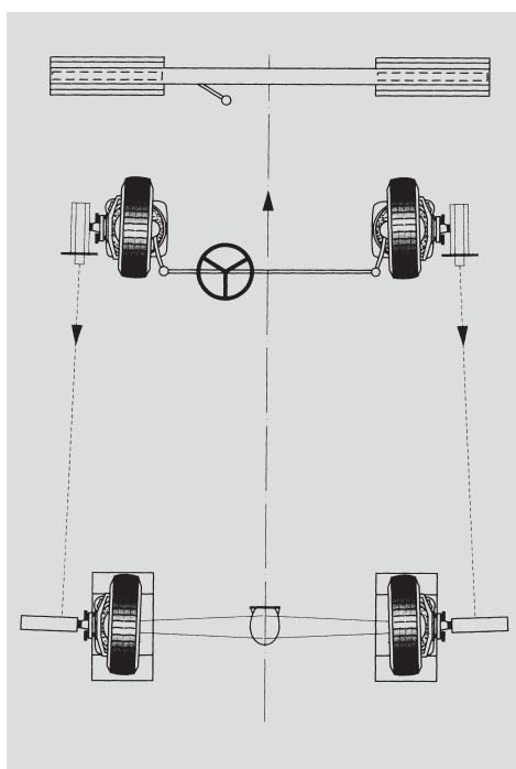
ZASADA DZIAŁANIA OPTYCZNYCH STANOWISK POMIAROWYCH. Z LEWEJ SYSTEM WYKORZYSTUJĄCY SKUPIONE ŚWIATŁO TRADYCYJNYCH ŻARÓWEK. Z PRAWIEJ URZĄDZENIE WYPOSAŻONE W GŁOWICE LASEROWE
